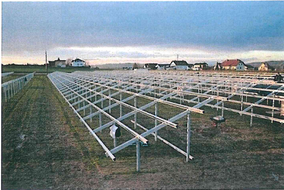
Rysunek 4. Szkielety przed montażem paneli, farma solarna NIENBURG 4 MW (Niemcy) (Remor Solar)
