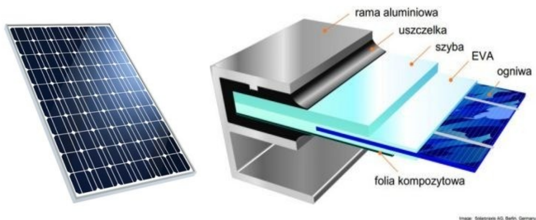
Rysunek 2. Pojedynczy moduł fotowoltaiczny oraz jego przekrój.
