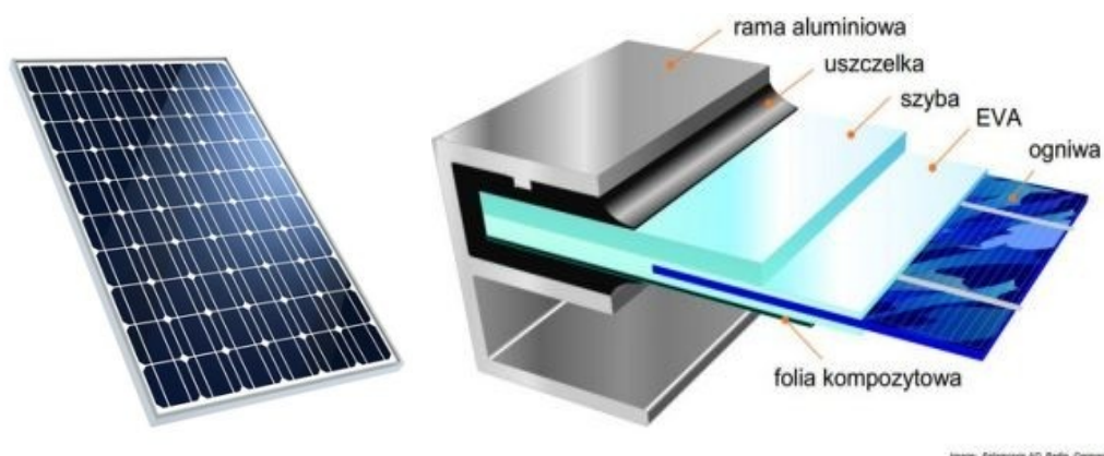
Rysunek 2. Pojedynczy moduł fotowoltaiczny oraz jego przekrój.
